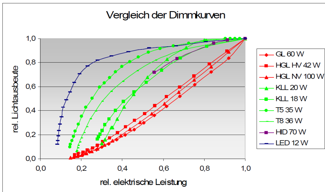
Bild 12. Lichtausbeute in Abhängigkeit von der elektrischen Leistung beim Dimmen
