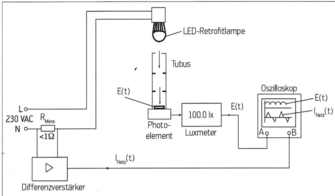
Bild 8. Schema zur Messung der Lichtwelligkeit
