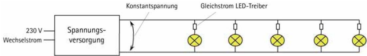
Bild 2. LEDs mit Konstantspannungs-Treiber
