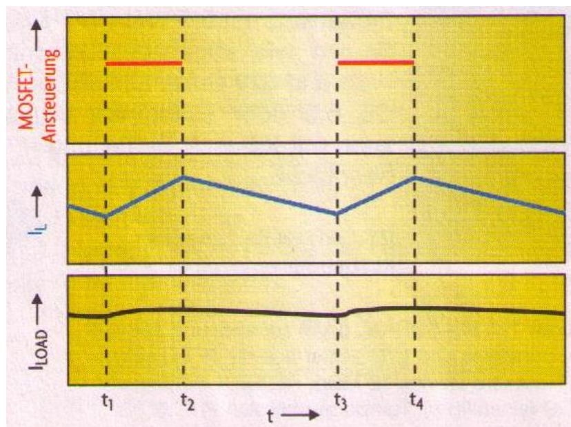
Bild 7. Signaldiagramm zur analogen LED-Stromregelung
