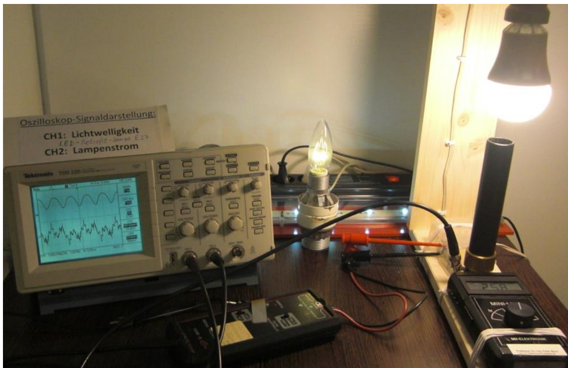
Bild 9. Messaufbau zur Bestimmung der Lichtwelligkeit mit einem Luxmeter und einem digitalen Speicheroszilloskop (DSO). Auf dem Bildschirm sieht man oben die Lichtwelligkeit des Lichtstroms und darunter den gravierend nichtsinusförmigen Netzstrom der Retrofitlampe.
