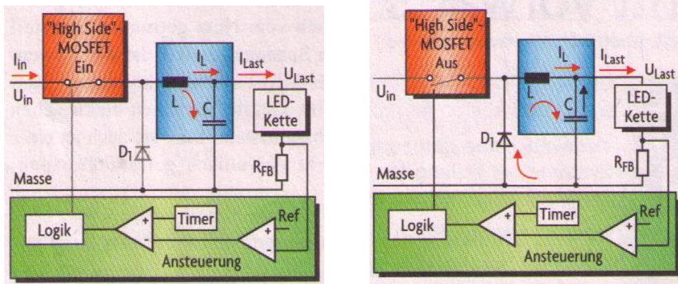
Bild 6. Arbeitsweise einer analogen LED-Stromregelung:
