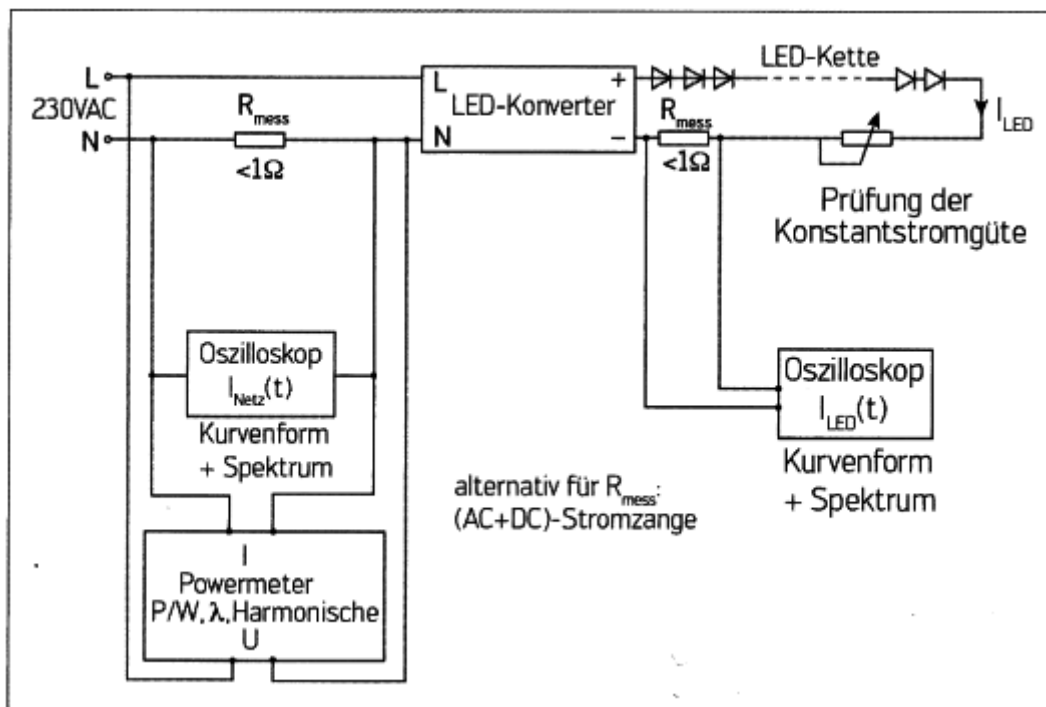
Bild 11. Schaltungsaufbau zur Untersuchung von LED-Konvertern
