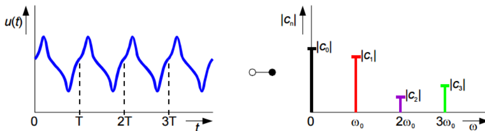
Bild 10. Darstellung der Lichtwelligkeit im Zeit- und Frequenzbereich
