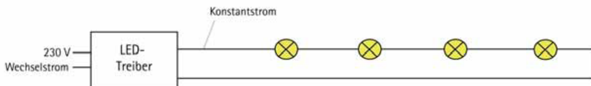
Bild 1. LEDs mit Konstantstrom-Treiber
