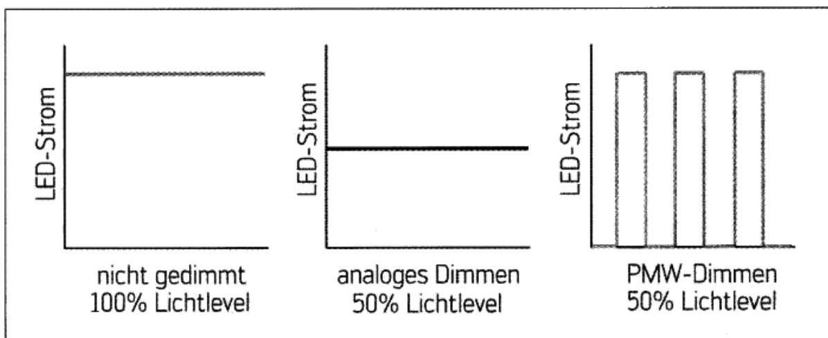
Bild 4. Analoges und PWM-Dimmen
