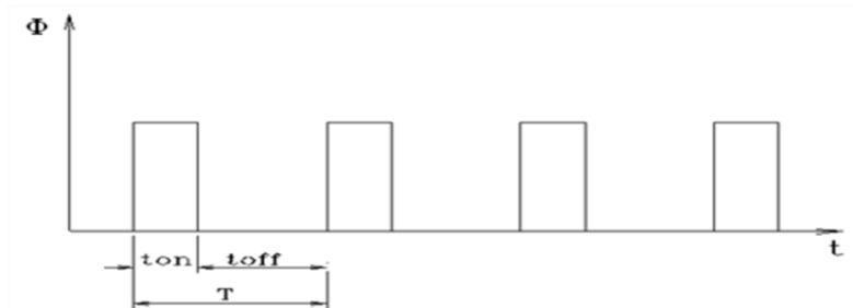
Bild 5. PWM-Verfahren: Signaldiagramm des zeitlichen Verlaufs des Lichtstroms
